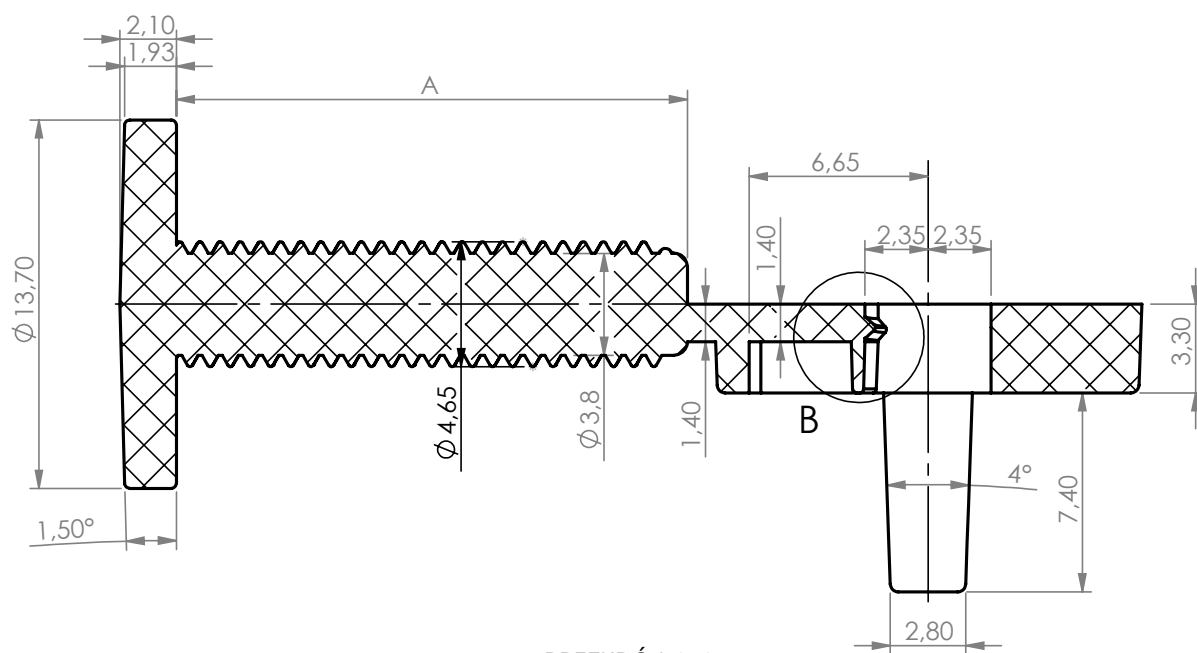
PRZEKRÓJ A-A
